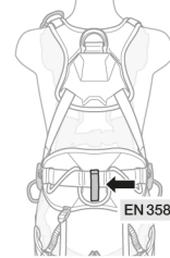
6d. Rear restraint attachment point Point d'attache arrière de retenue
