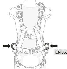
6c. Waistbelt side attachment points Points d'attache latéraux de ceinture
